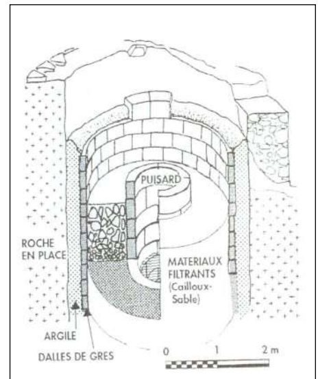
Figure de droite : Schéma d'une citerne filtrante Source : Bulletin communal Mairie d'Urbeis
